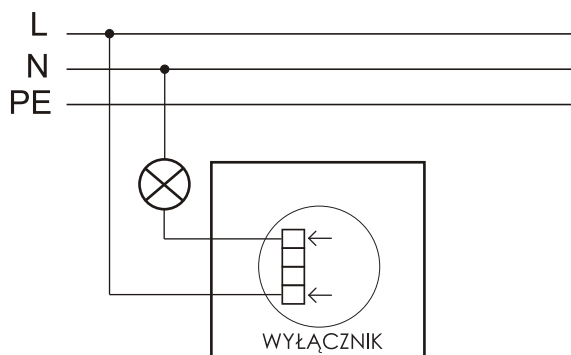
Schemat instalacji wyłącznika chwilowego (dzwonkowego).
